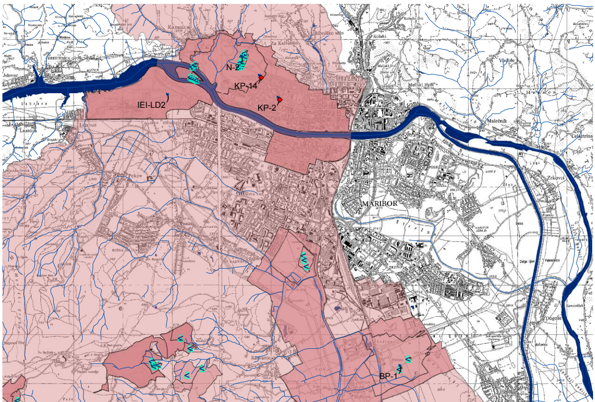
Slika 4: Pregled mest vzorčenja podzemne vode z ugotovljeno prisotnostjo atrazina
