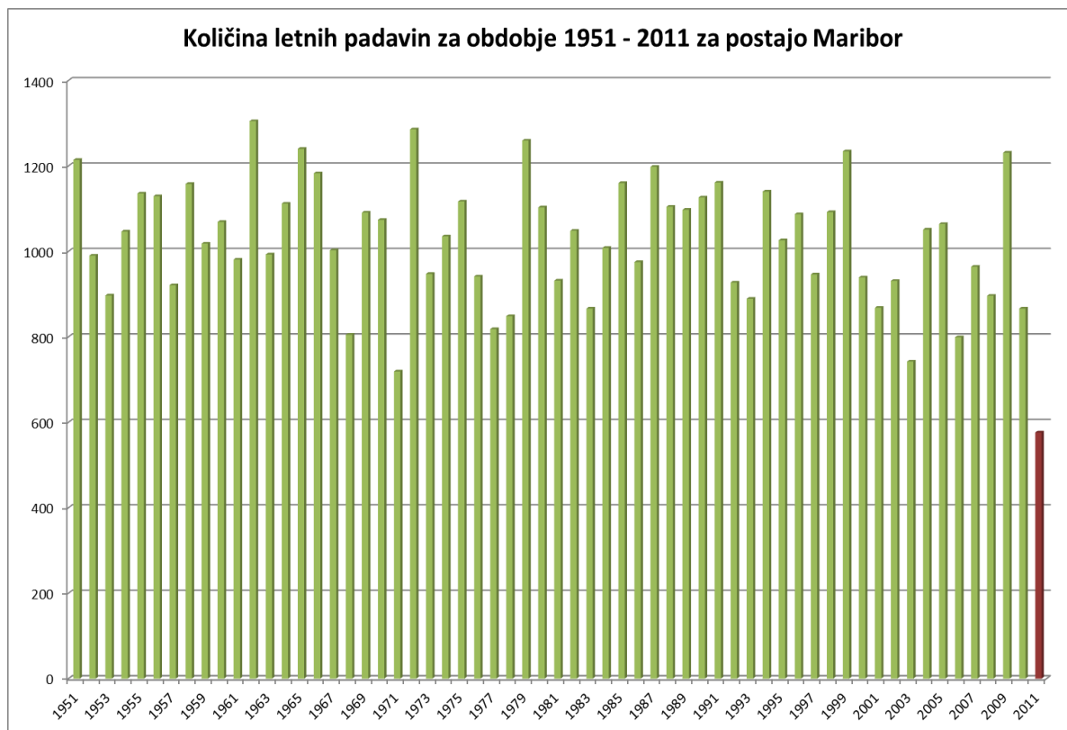
Slika 3: Količina letnih padavin za postajo Maribor-Tabor v obdobju od leta 1951 do 2011 (Vir: IEI)
