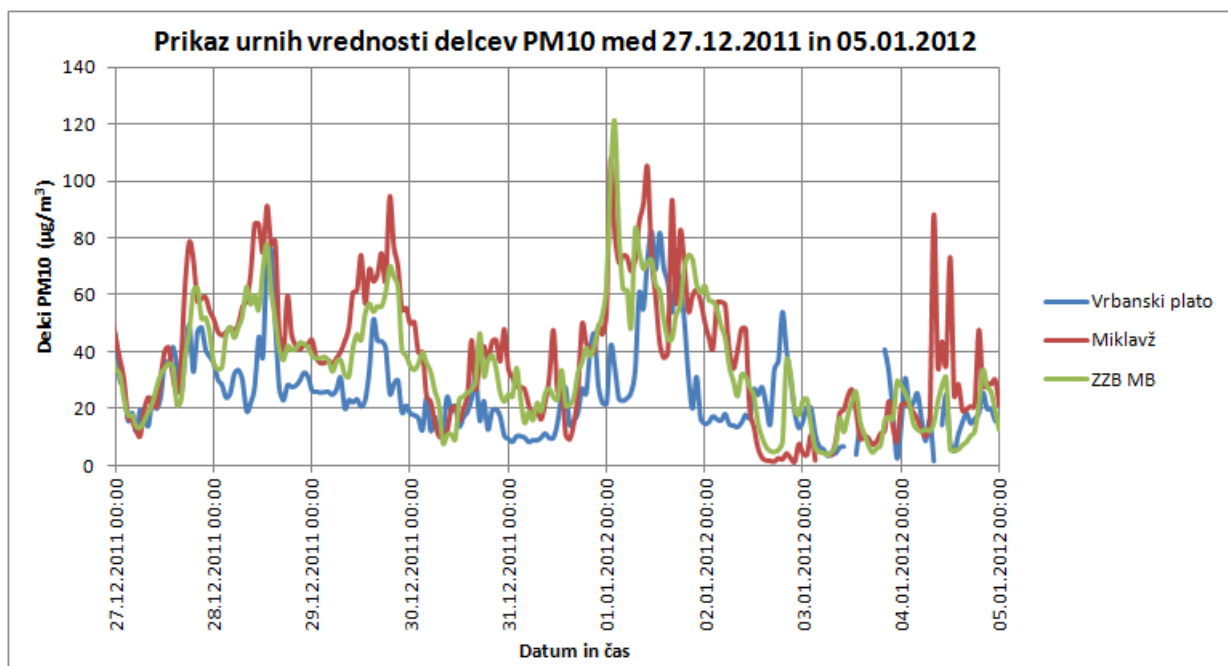
Slika 2: Prikaz urnih vrednosti delcev PM10 na prehodu v novo leto; mejna dnevna vrednost je 50 \mu\text{g}/\text{m}^3 (Vir: ZZV MB)
