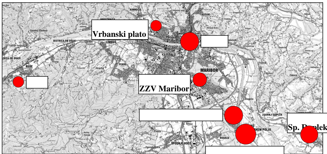
Slika 1: Srednje mesečne koncentracije delcev PM10 v decembru 2011 (Vir: ZZV MB)
