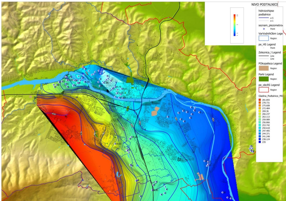
Slika 6: Gladina podzemne vode na obravnavanem območju Vrbanski plato, Dravsko polje
