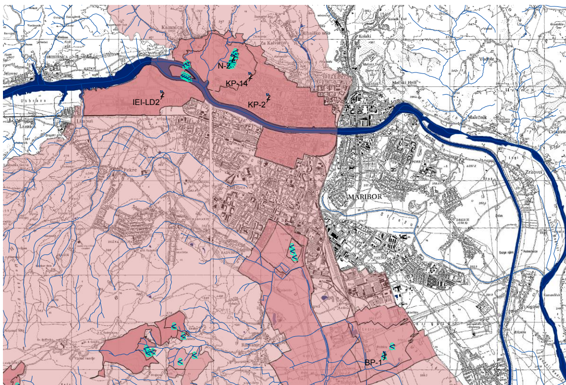
Slika 5: Pregled mest vzorčenja podzemne vode z ugotovljeno prisotnostjo halogeniranih lahkohlapnih ogljikovodikov (LKCH)
