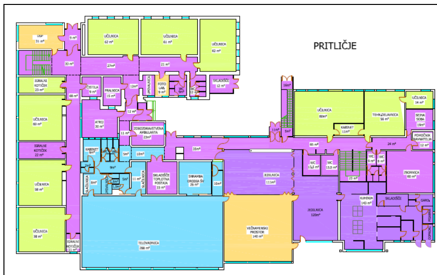
Slika 3: Tloris pritličja OŠ Ludvika Pliberška Maribor.
