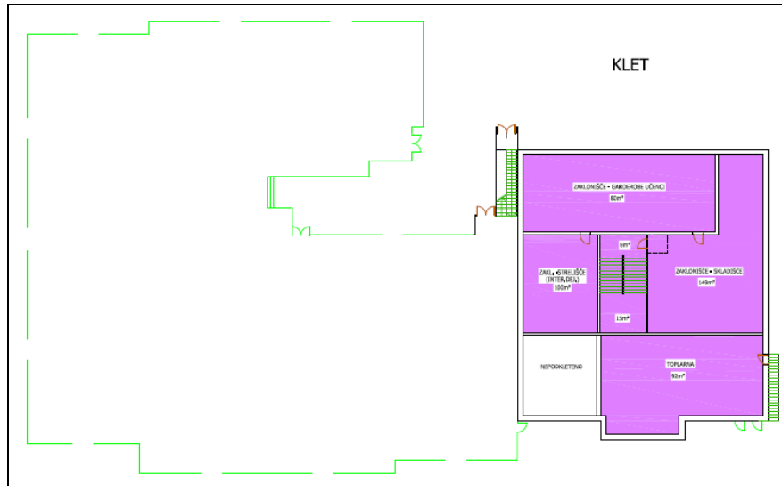
Slika 2: Tloris kleti PŠ Ludvika Pliberška Maribor.
