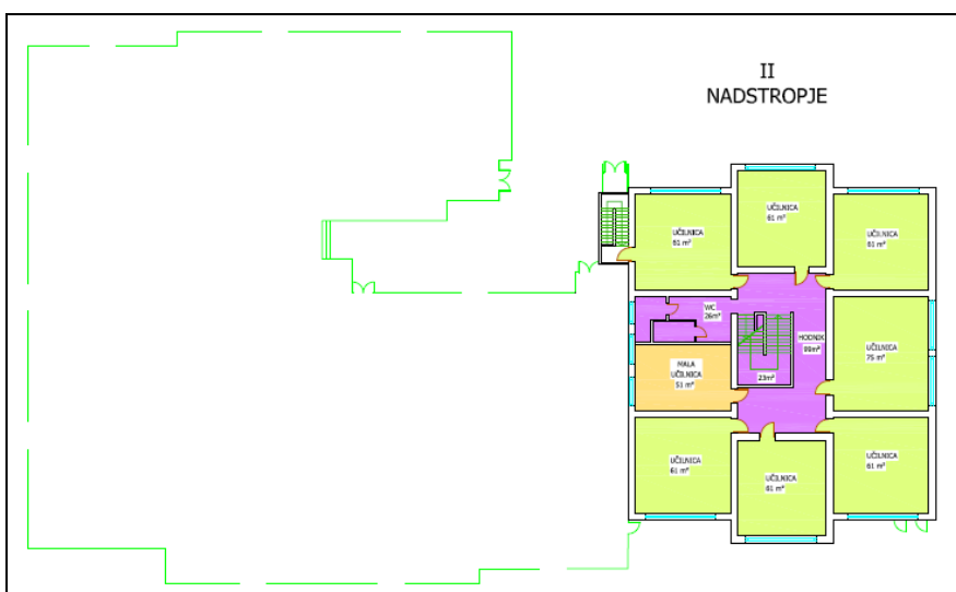
Slika 5: Tloris drugega nadstropja OŠ Ludvika Pliberška Maribor.
