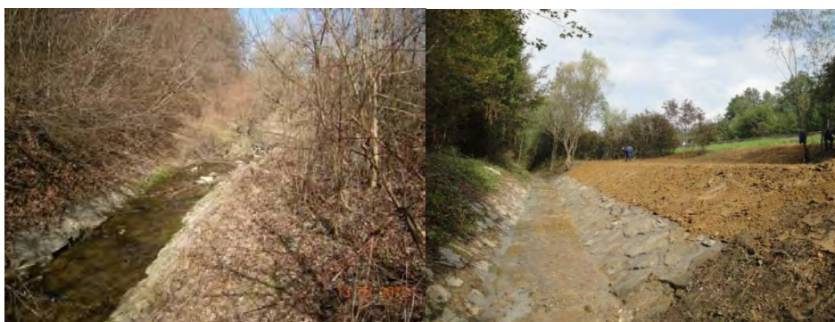
Slika 12 : pred in po sanaciji brežine in kamnitih oblog
