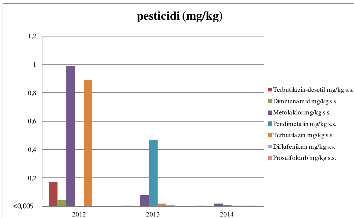
Slika 5: Vsebnosti najdenih pesticidov v zemljinah
