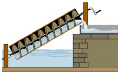
Slika 1: Princip Arhimedovega vijaka (Spletna stran SMART Technologies ULC)
