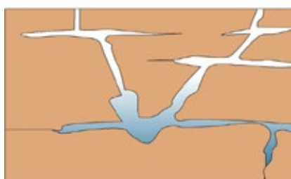
Slika 2: Različni tipi poroznosti: a) medzrnska, b) kanalska oziroma kraška in c) razpoklinska (Spletna stran Colorado Geological Survey)
