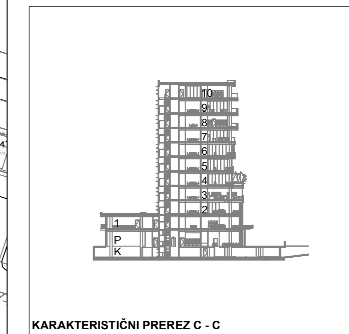
KARAKTERISTIČNI PREREZ C - C
