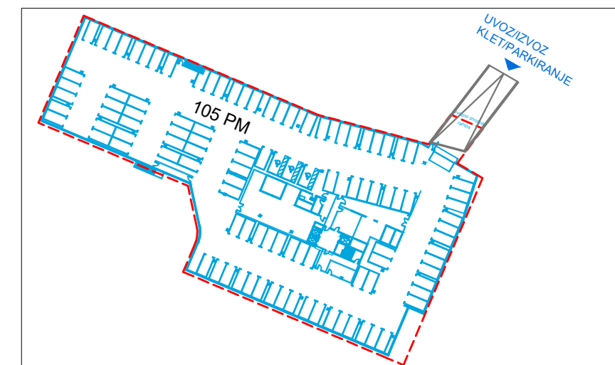
SHEMATSKI PRIKAZ KLETNE ETAŽE - GARAŽE - OBJEKT 2 M 1:1000
