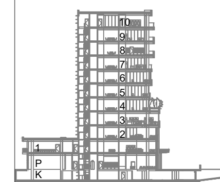
KARAKTERISTIČNI PREREZ C - C M 1:1000
