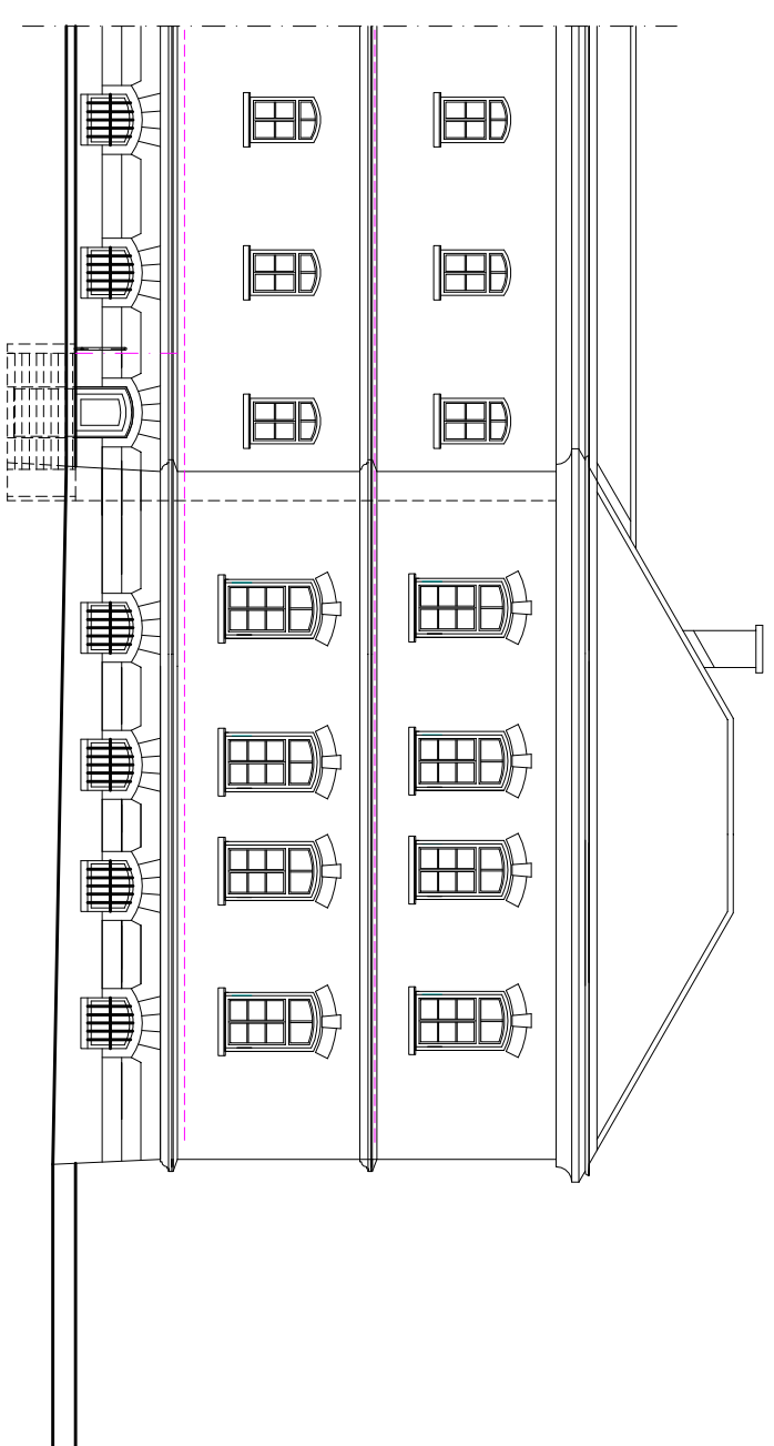
SEVERNA FASADA
