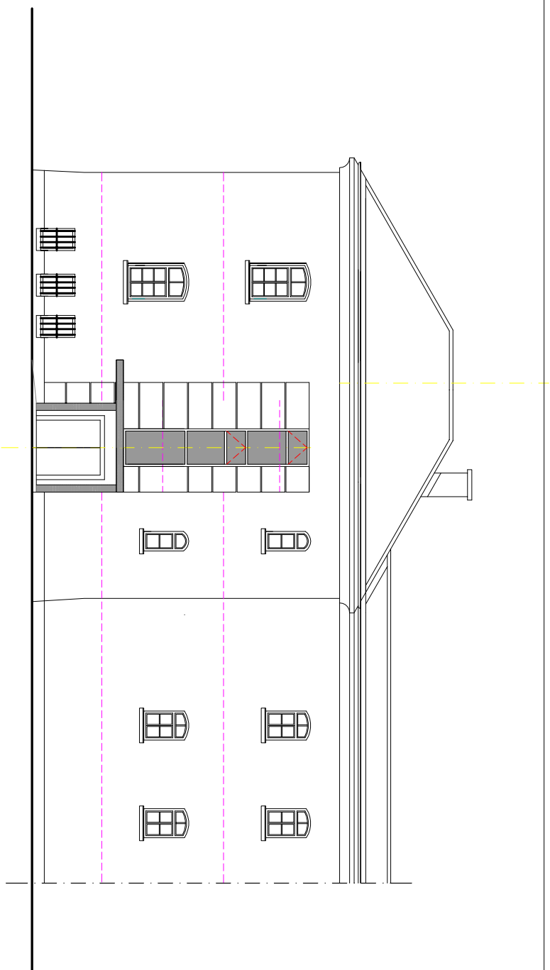
JUŽNA FASADA
